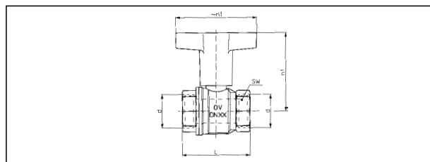
арт. № 107 71 03-16 (Ду 10 до Ду 50) Маховик пластмассовый, удлиненный
