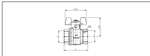
арт. № 107 61 03-10 (Ду 10 до ДуN 25) Маховик алюминиевый
