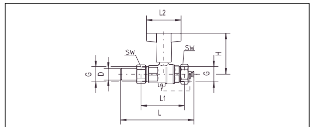
арт. № 106 66 04- 10 (Ду 15 до Ду 32) Маховик пластмассовый, удлиненный
