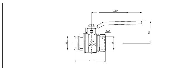
арт. № 107 62 03-10 (Ду 10 до ДуN 32) Рукоятка рычажная из оцинкованной стали в пластмассовой оболочке
