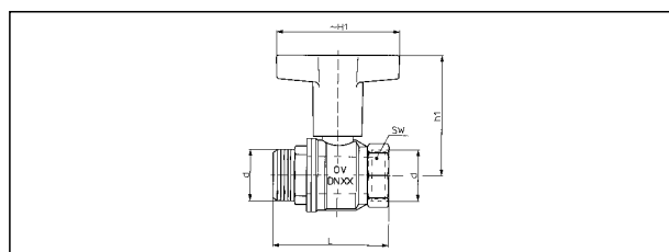
арт. № 107 73 03-10 (Ду 10 до Ду 32) Маховик пластмассовый, удлиненный
