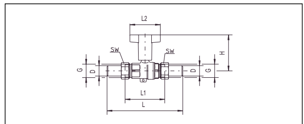
арт. № 106 56 04- 10 (Ду 15 до Ду 32) Маховик пластмассовый, удлиненный
