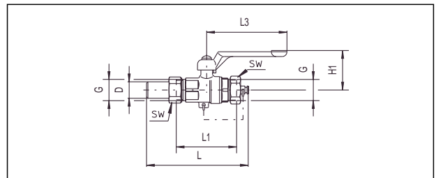
арт. № 106 65 04- 10 (Ду 15 до DN 32) Маховик алюминиевый
