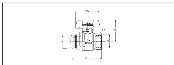
арт. № 107 63 03-10 (Ду 10 до Ду 25) Маховик алюминиевый
