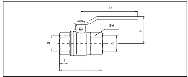
арт. № 107 65 02- 16 (Ду 6 до Ду 50) Рукоятка рычажная из оцинкованной стали в пластмассовой оболочке
