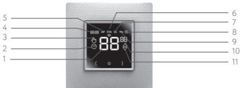
Рис. 26. Индикация прибора
