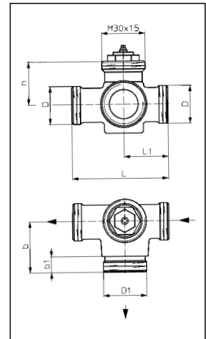
правостороннее присоединение
